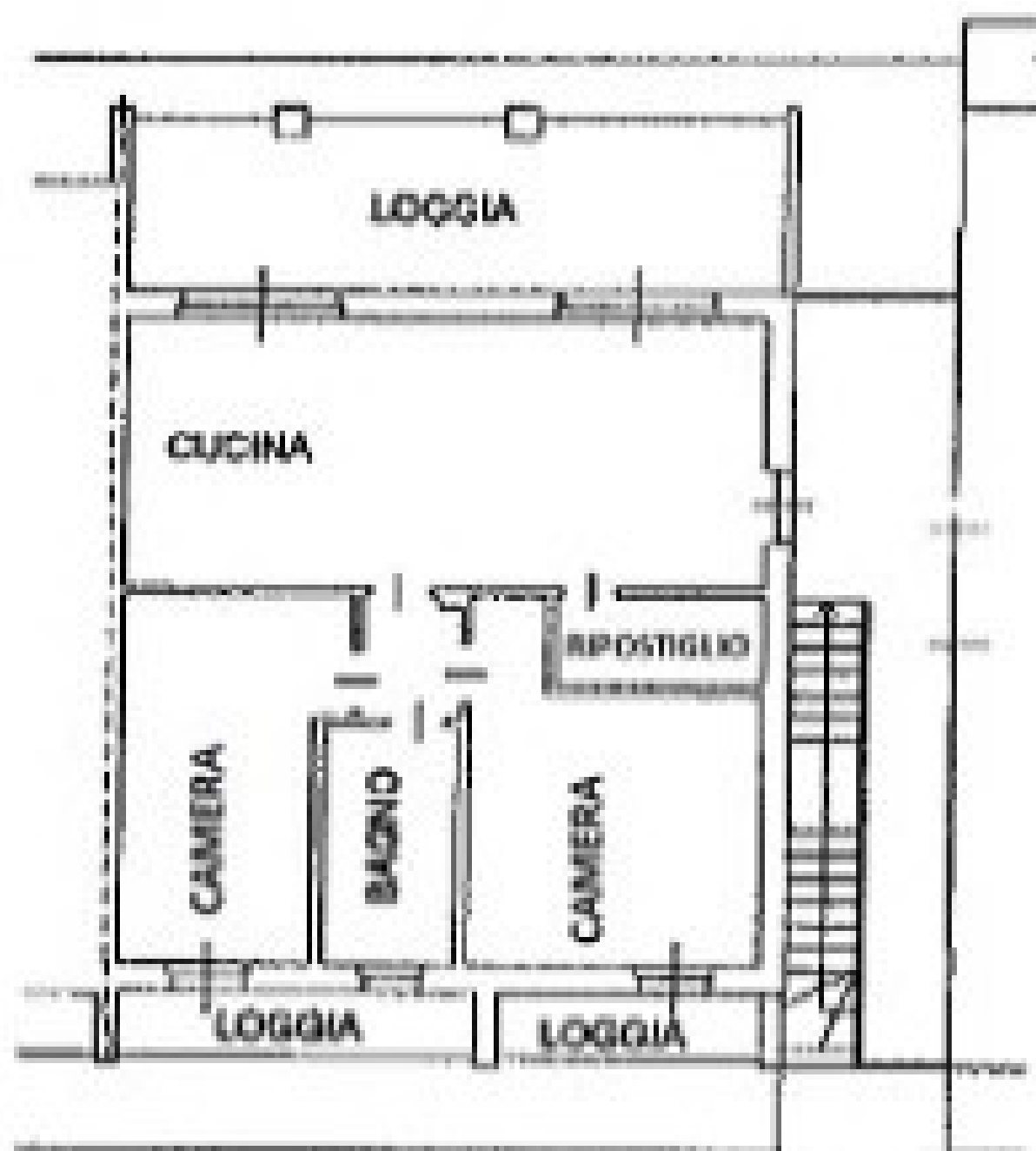
PIANO PRIMO
